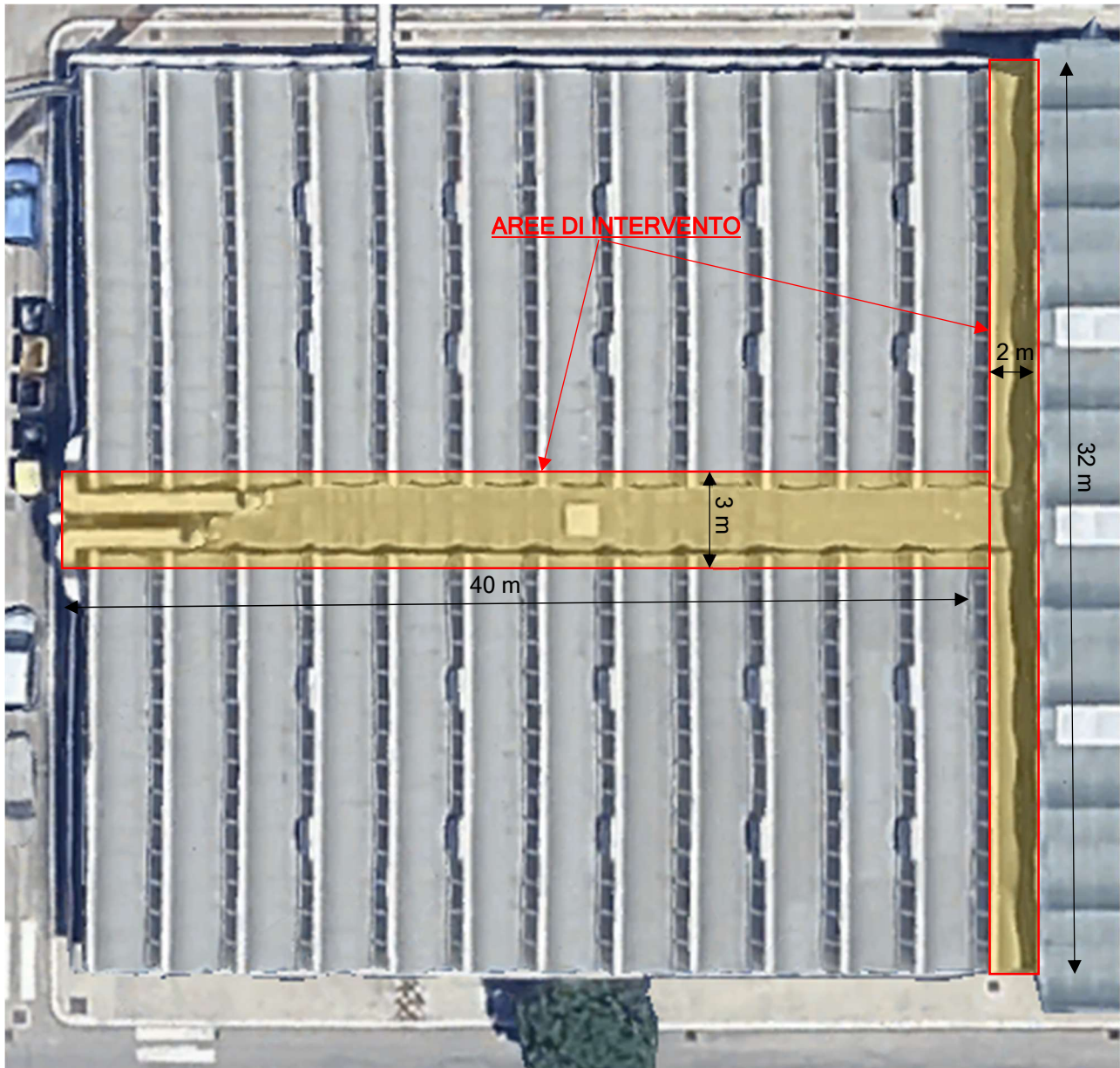
Figura 2 – Area di intervento copertura lato Ponente
