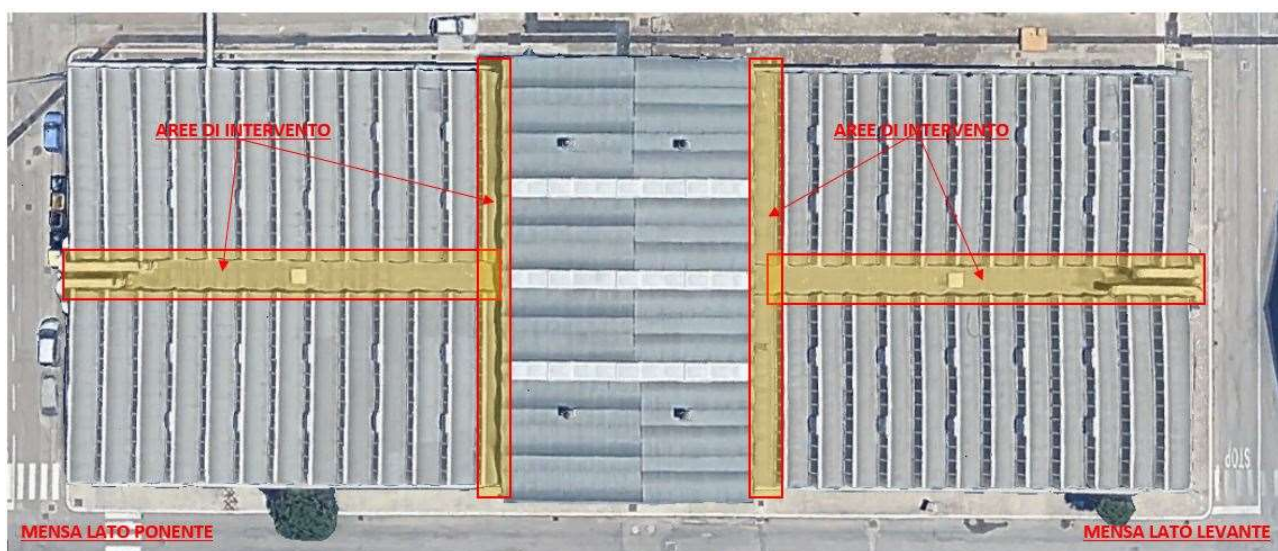
Figura 1 – Vista complessiva della copertura con indicazione delle aree di intervento
